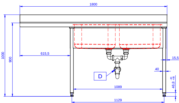
Zij aanzicht
